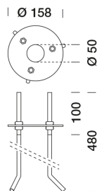
8950075 Tie-rod Ø 158 x D. 480
