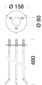
8950155 Tie-rod
